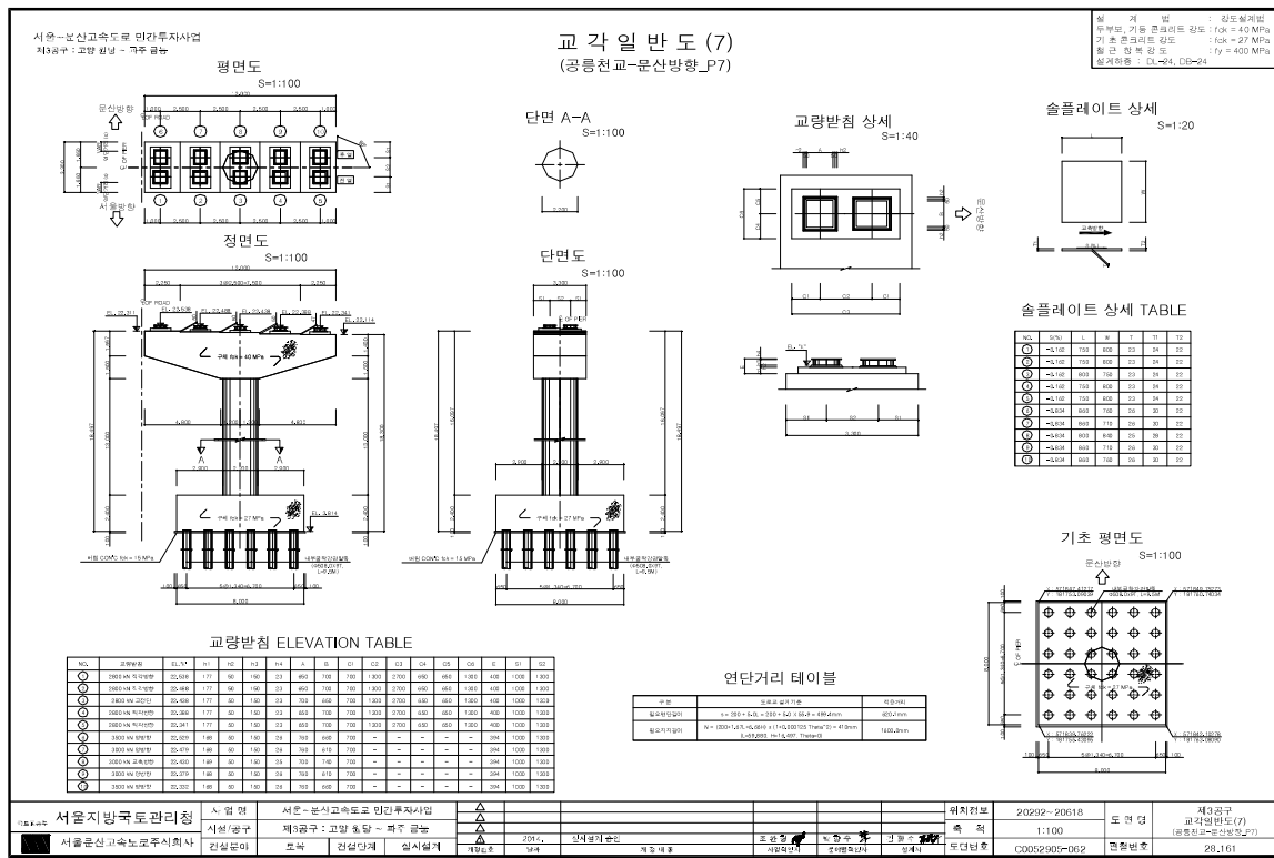
【그림 35.1.7】 교각 일반도
